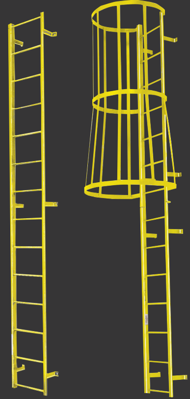
14 Rung Standard F14S
